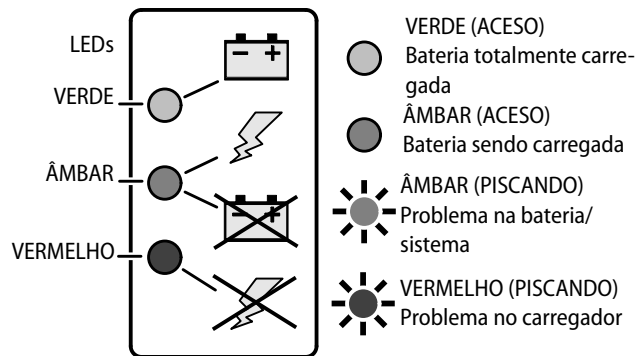
Figura 3-12. Adesivo do Carregador dos LEDs Indicadores
