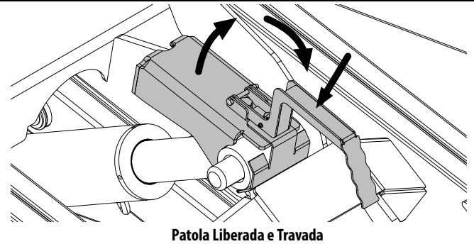
Figura 3-16. 3248RS/10RS - Braço Tipo Tesoura - Patola de Segurança
