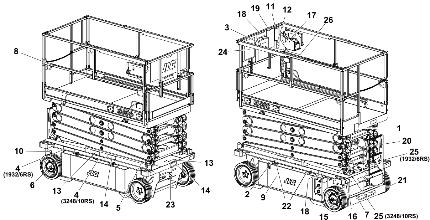
Figura 5-4. Instalação dos Adesivos da Máquina - Todas as Máquinas
