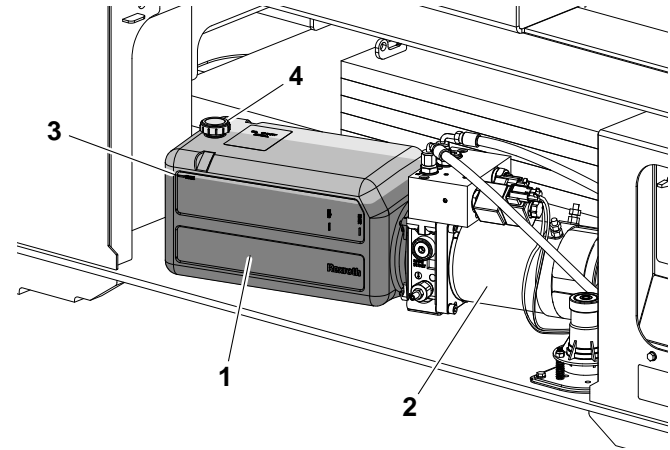
Figura 5-1. Procedimento de Verificação do Óleo Hidráulico - Todas as Máquinas
