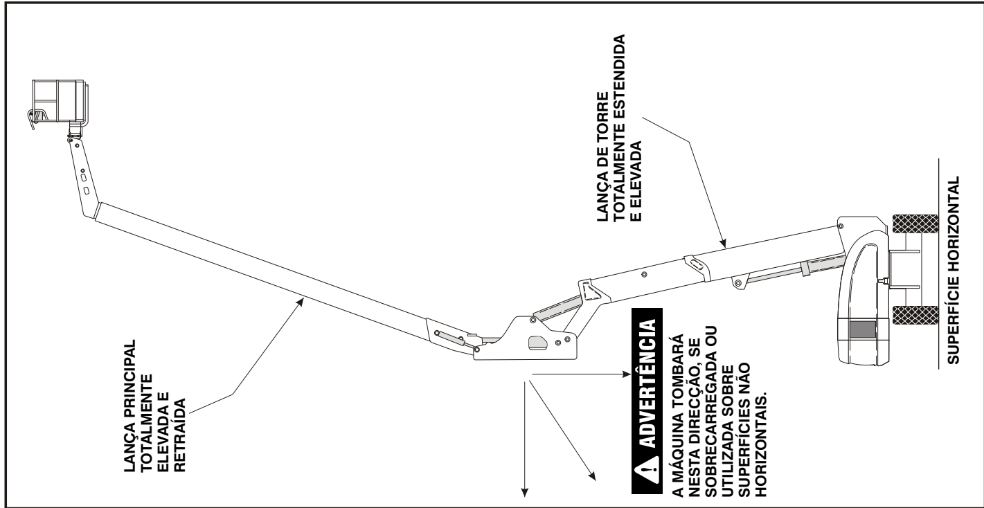
Figura 4-3. Posição da menor estabilidade posterior (Folha 2 de 2)
