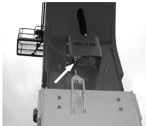
Figura 2-8. Interruptor de fim-de-curso horizontal da lança de torre
